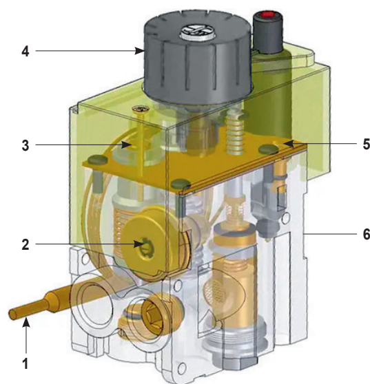
Рис. 11. Газовый блок TGV 307
