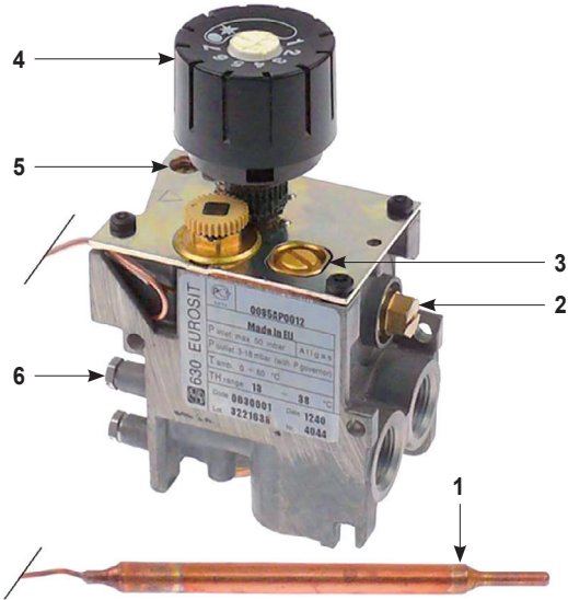
Рис. 11. Газовый блок 630 EUROSIT
