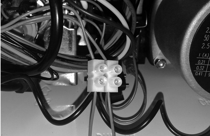
Рис. 5. Доступ к клеммной колодке
