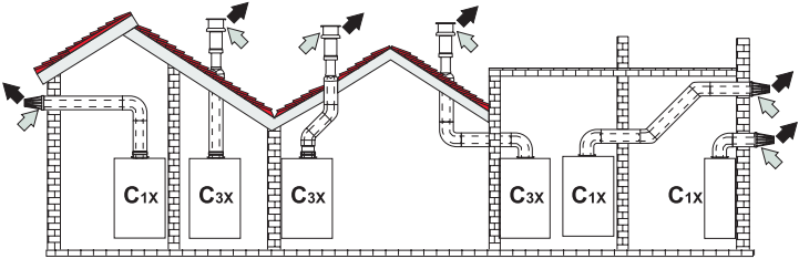
Рис. 7. Пример установки коаксиального дымохода (воздух/дым)
