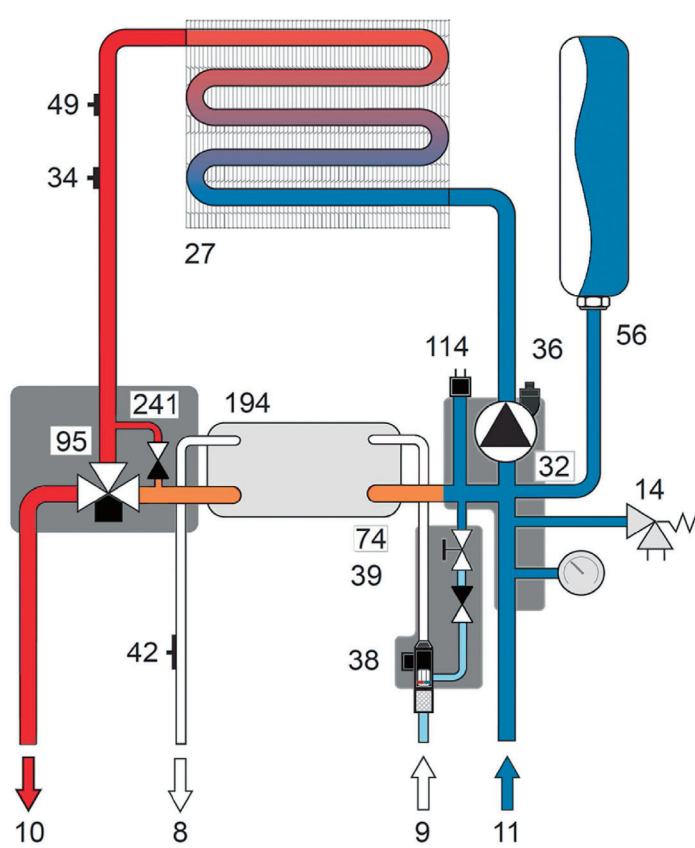
Рис. 14 Гидравлический контур
