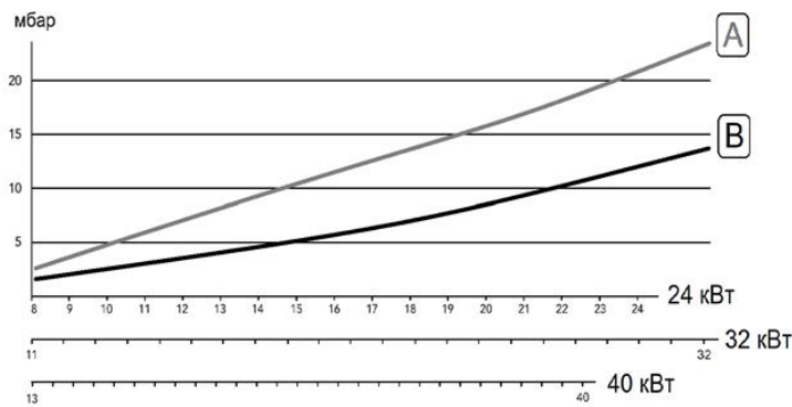
A – сжиженный газ B – природный газ
