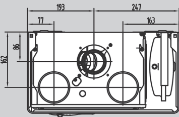
VITABEL C24
