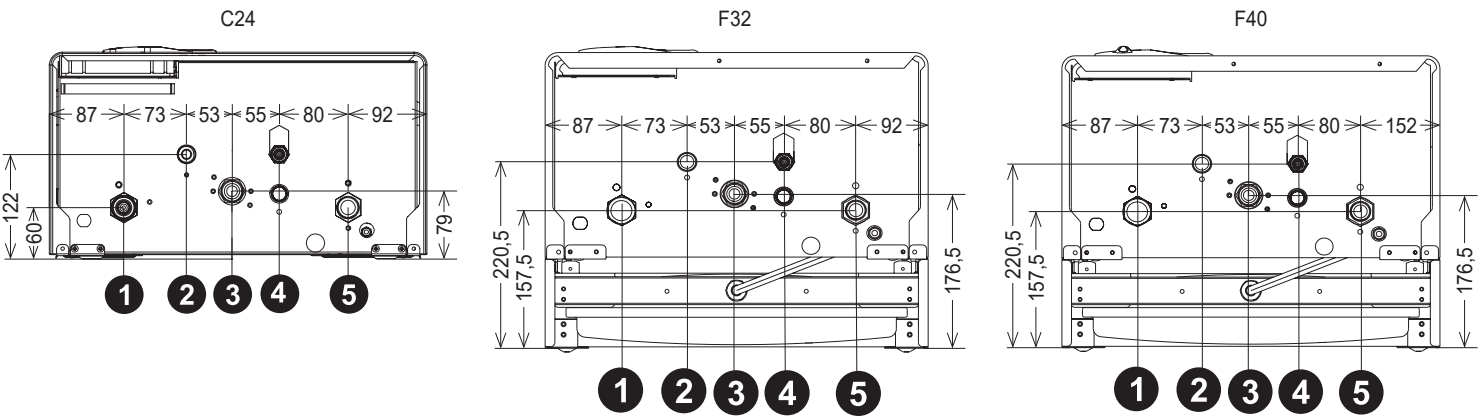
1) подача в систему отопления; 2) выход горячей воды; 3) вход газа; 4) вход холодной воды; 5) возврат из системы отопления.
