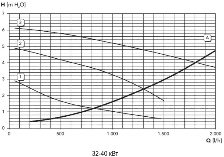
A – потери напора в котле; 1, 2, 3 – скорость циркуляционного насоса
