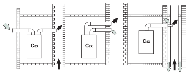
Рис. 14. Примеры подсоединения к дымоходам
