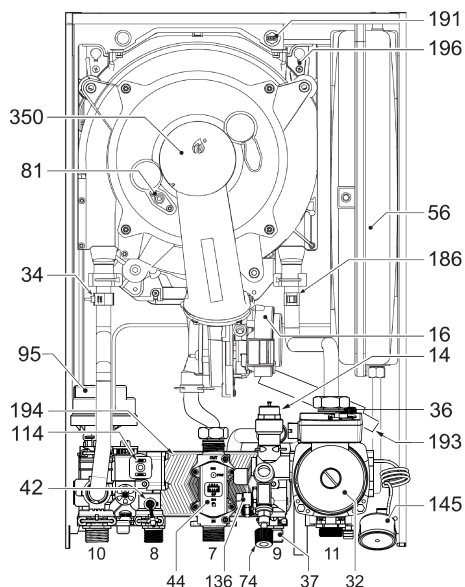
Рис. 40. Конструкция
