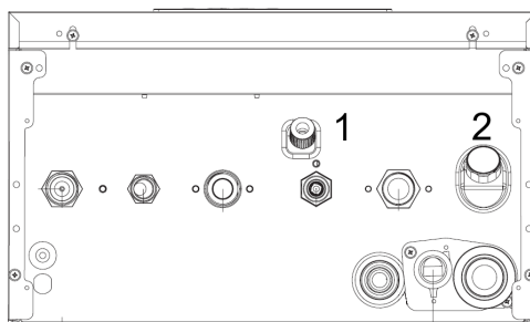
Рис. 16. Ручка заполнения системы
