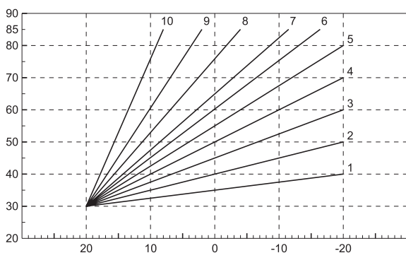
Рис. 14. Компенсационные кривые
