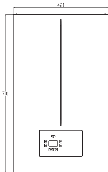
Рис. 36. Вид спереди
