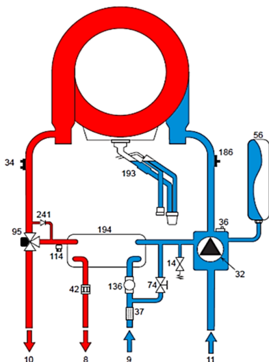
Рис. 41. Гидравлическая схема
