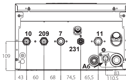
Рис. 35. Вид снизу
