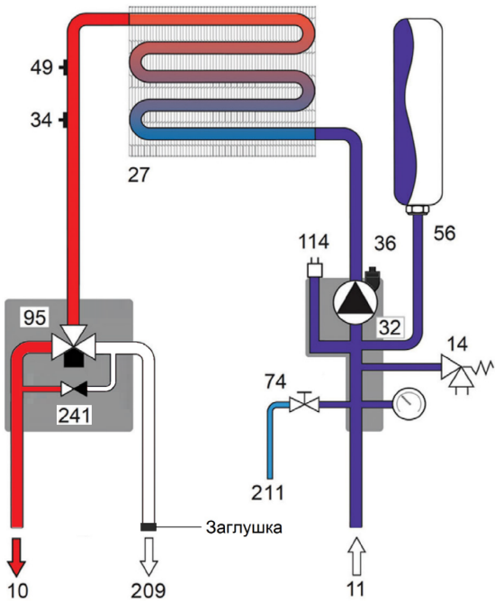
Рис. 18. Отопительный контур
