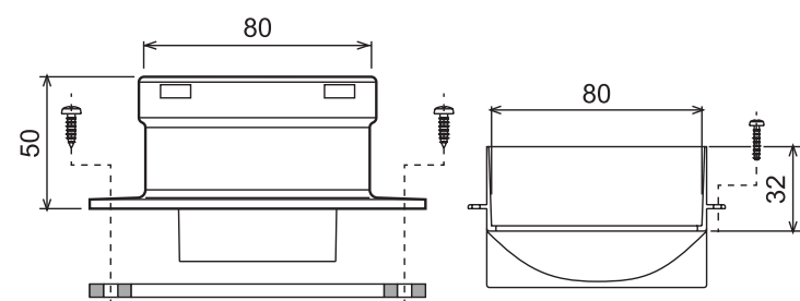
Рис. 11. Начальные элементы для раздельного дымохода
