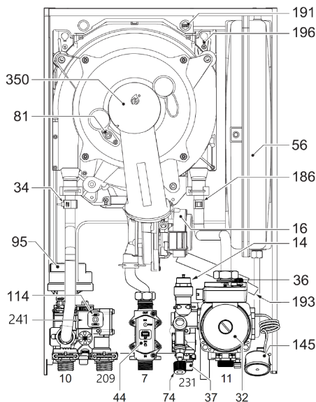
Рис. 40. Конструкция
