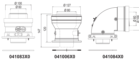
Рис. 21а. Стартовые аксессуары для коаксиального дымохода
