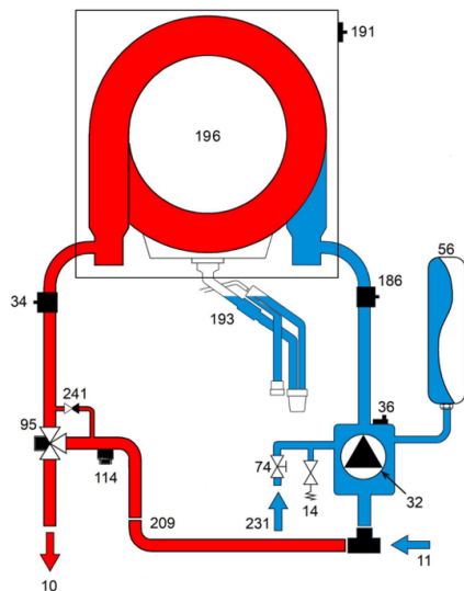
Рис. 41.а Гидравлическая схема. Без бойлера
