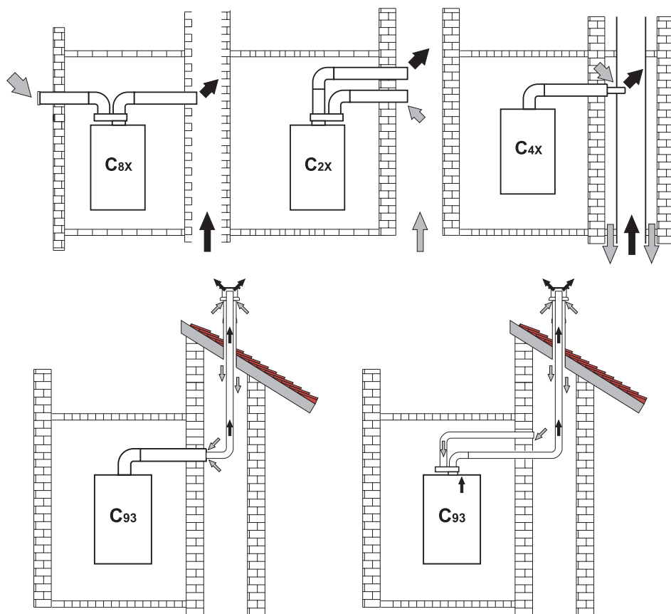
Рис. 26. Примеры присоединения к коллективному дымоходу
