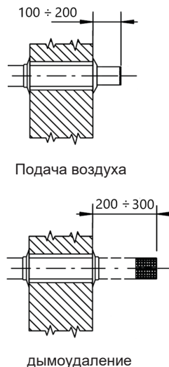
Рис.23б. "Вылет" труб раздельного дымохода
