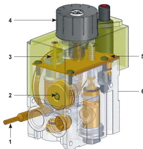
Рис. 11. Газовый блок TGV 307
