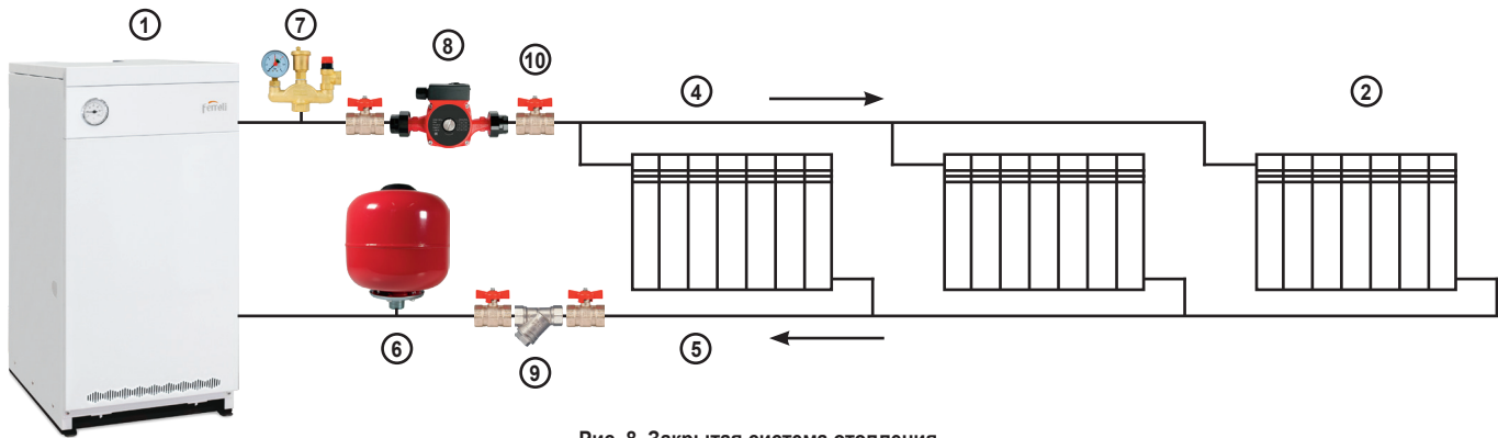
Рис. 8. Закрытая система отопления
