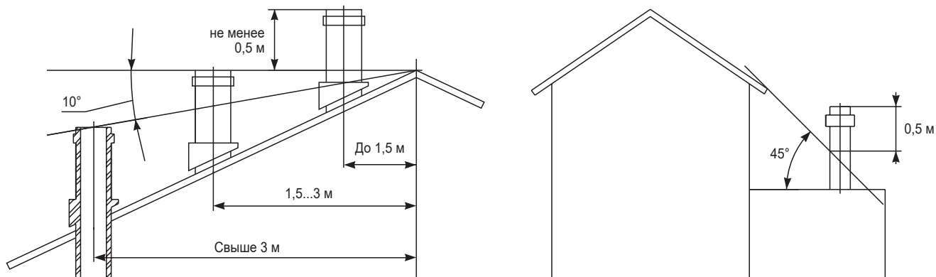
Рис. 6. Схема расположения дымовой трубы
