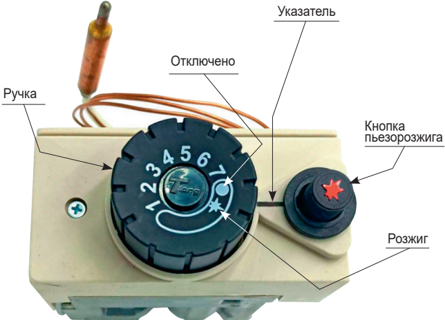
Рис. 9. Элементы управления на газовом блоке управления TGV 307
